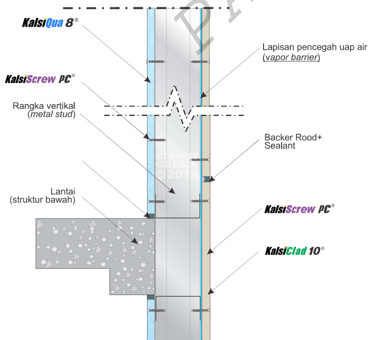
DETIL A-A
