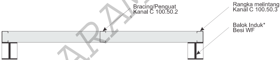
POTONGAN A-A
