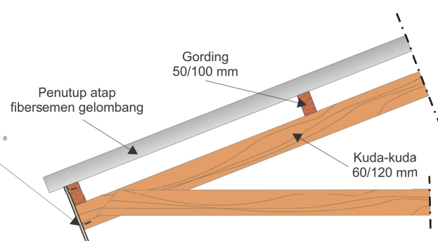
Gambar detail listplank pada posisi ujung atap (Penutup atap fibersemen gelombang)
