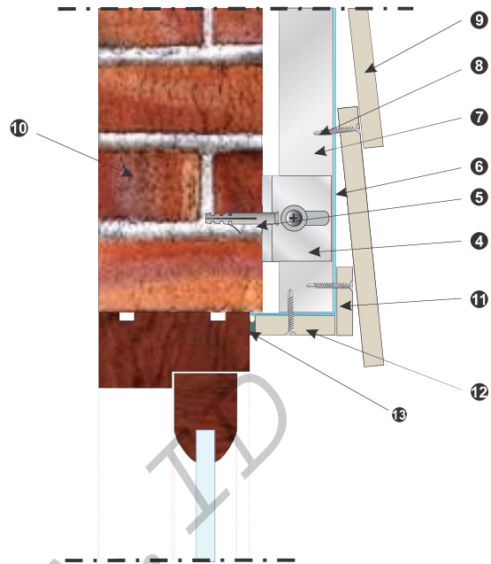
DETIL A
