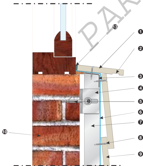
DETIL B
