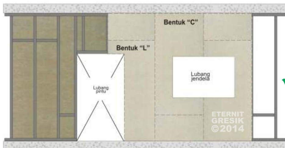
Pola pemasangan yang benar (pola zig-zag tipe 2)
