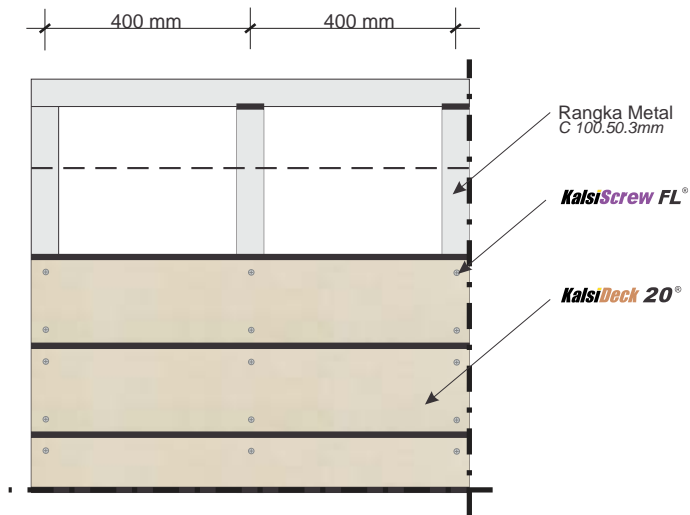
Gambar detil sistem lantai decking dengan rangka metal
