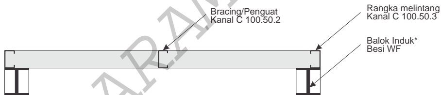
POTONGAN A-A
