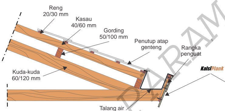
Gambar detail listplank pada posisi penutup talang (Penutup atap genteng)
