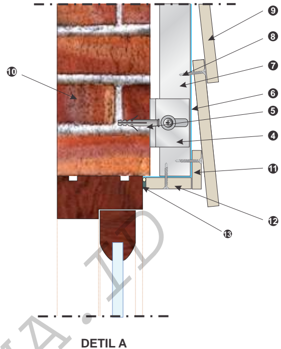
DETIL A
