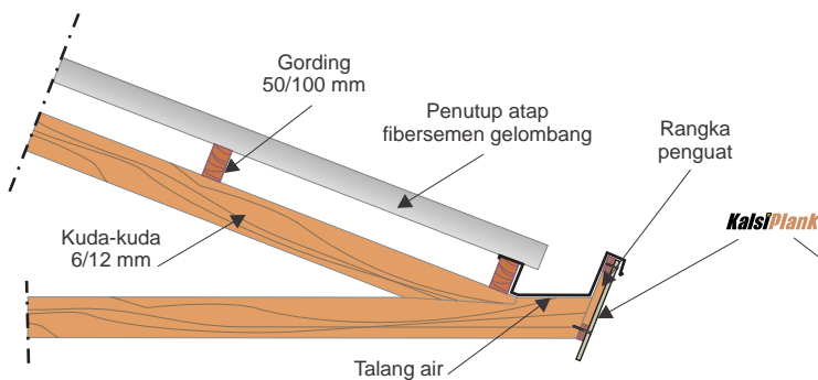
Gambar detail listplank pada posisi penutup talang (Penutup atap fibersemen gelombang)
