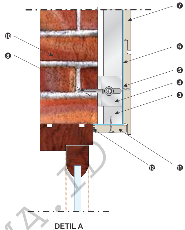
DETIL A (Sambungan kusen jendela bagian atas)
