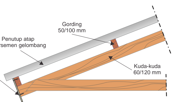
Gambar detail listplank pada posisi ujung atap (Penutup atap fibersemen gelombang)
